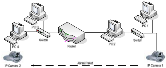
Gambar 2. Topologi Pengujian
